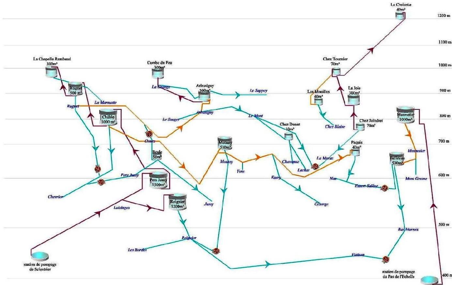
Figure 4: Schéma altimétrique du réseau en rive gauche de l'Arve.
